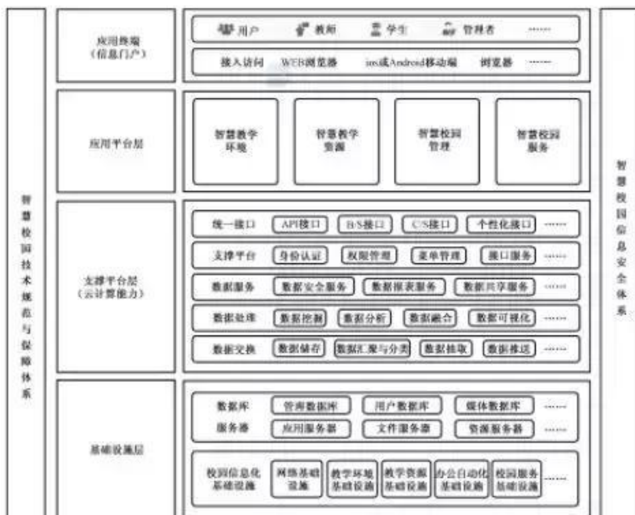
图1 智慧校园总体架构图
